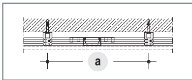
Расстояние между подвесами (дюбелями)
