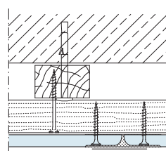
Продольный стык
