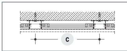
Межосевое расстояние основных профилей
